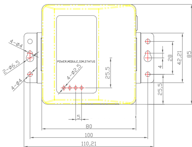
正视图
