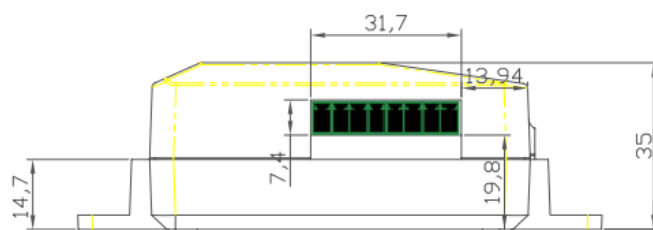
侧视图
