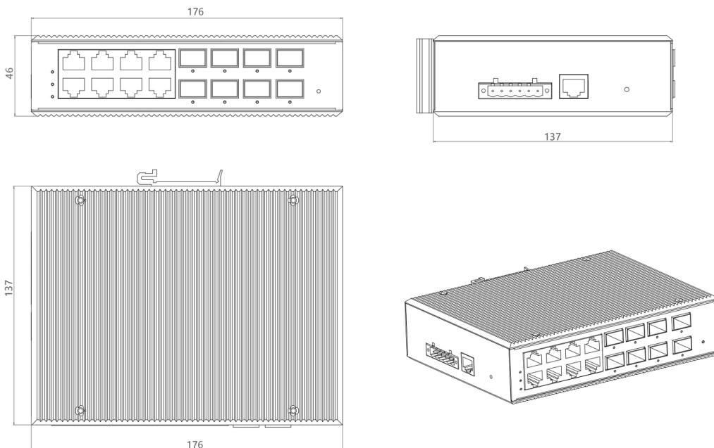
ISM5016 尺寸图
