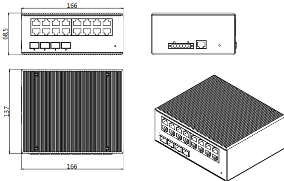
ISM5020D 尺寸图
