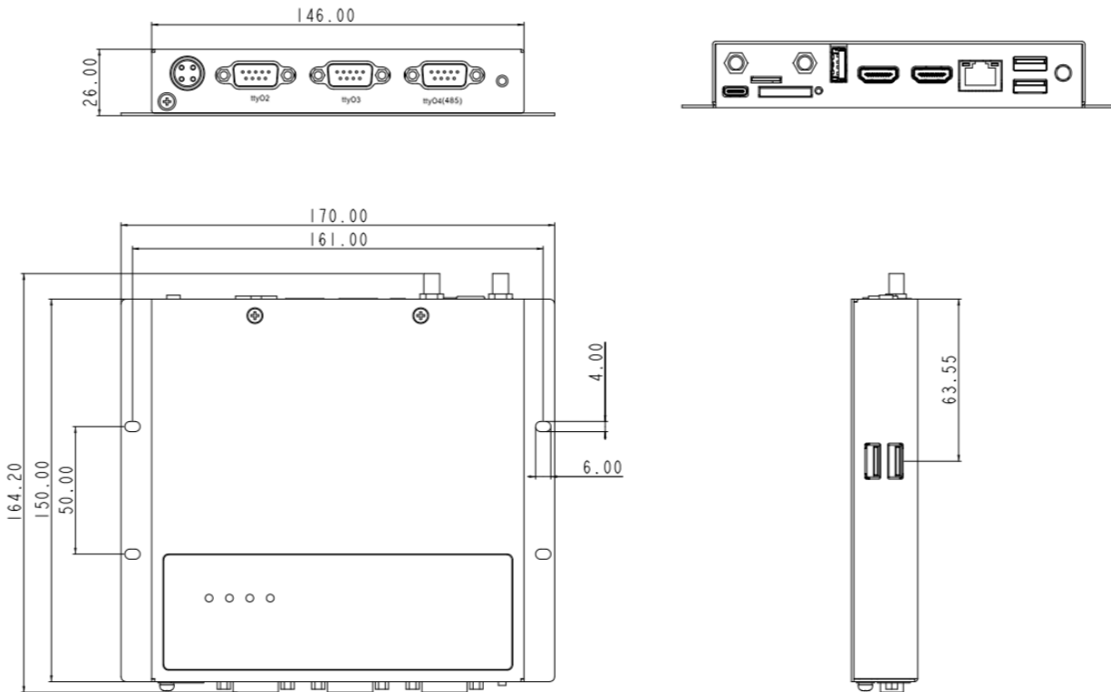
InBOX712产品尺寸图
