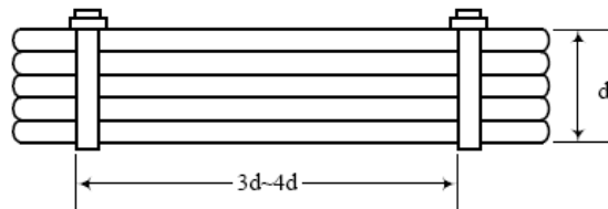
图 4-8 成束时的扎带
