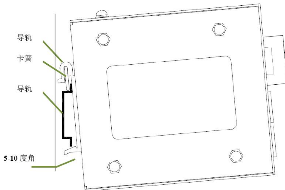
图 4-1 导轨式安装
